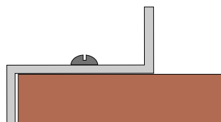
Kaderprofiel 20 * 40 * 20 mm.
