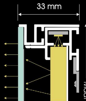
reflex standaard
