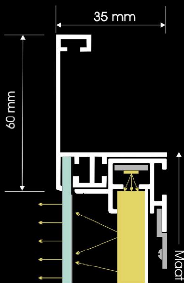
reflex passe-partout
